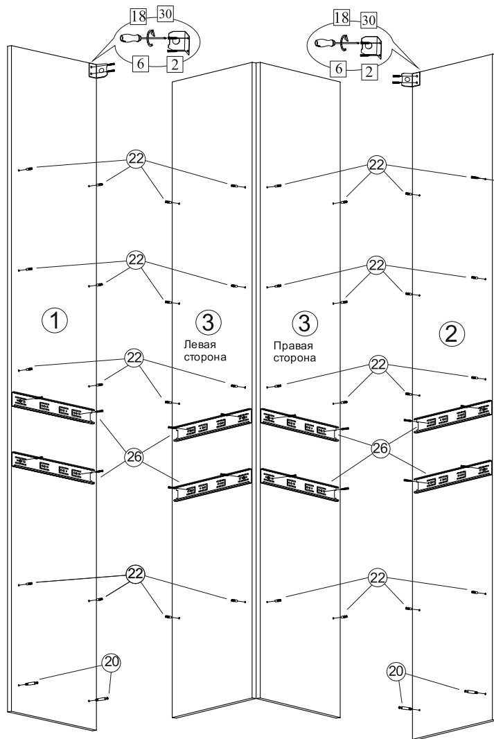
Рис.2 Монтаж фурнитуры на боковины и перегородку
