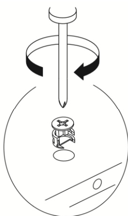
Рис.8 - Установка стяжки-полкодержателя
