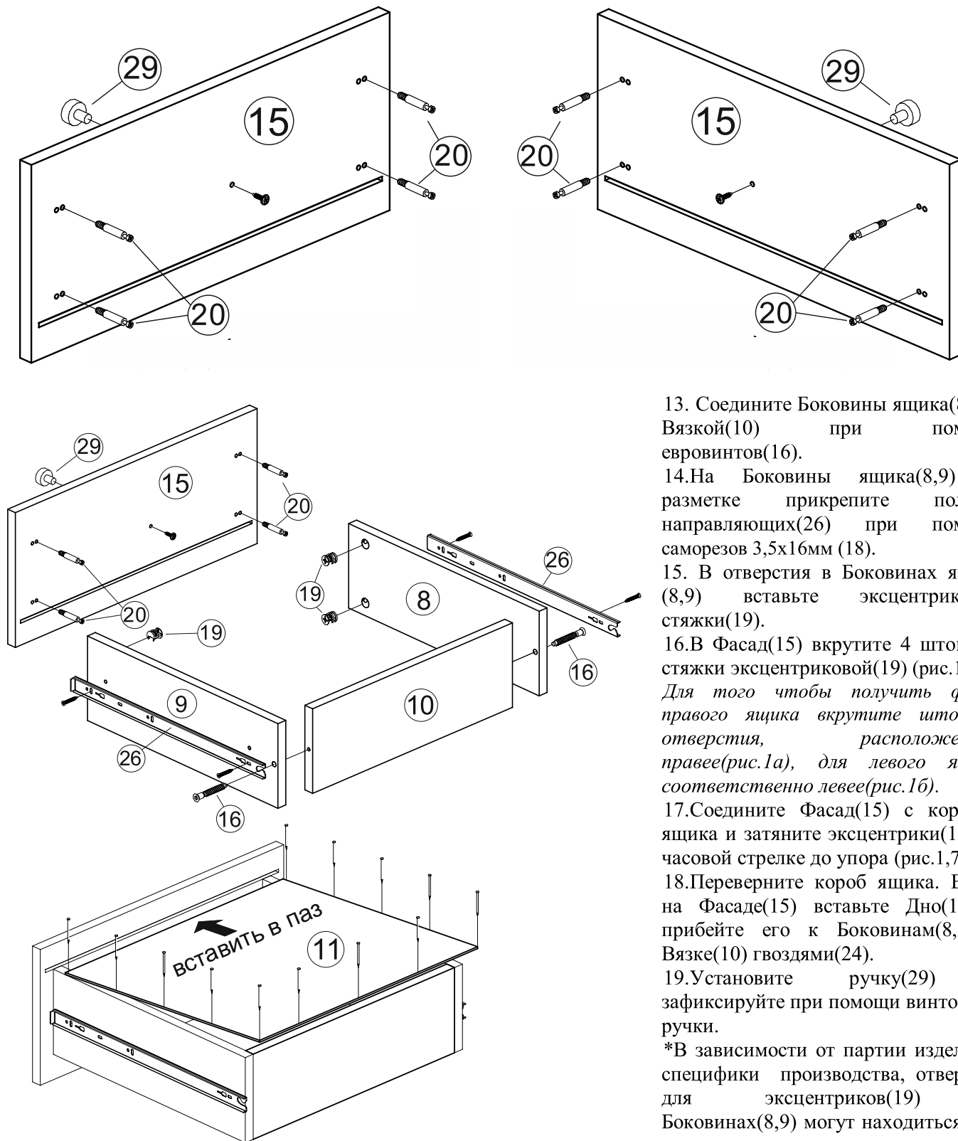
Рис.1а - Фасад правого ящика(2шт.)
