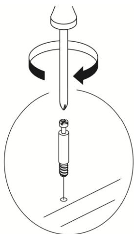
Рис.6 - Установка штока эксцентрика
