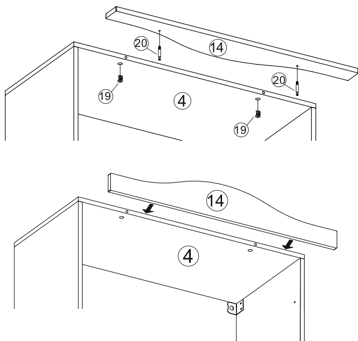
Рис.4 Монтаж Карниза
